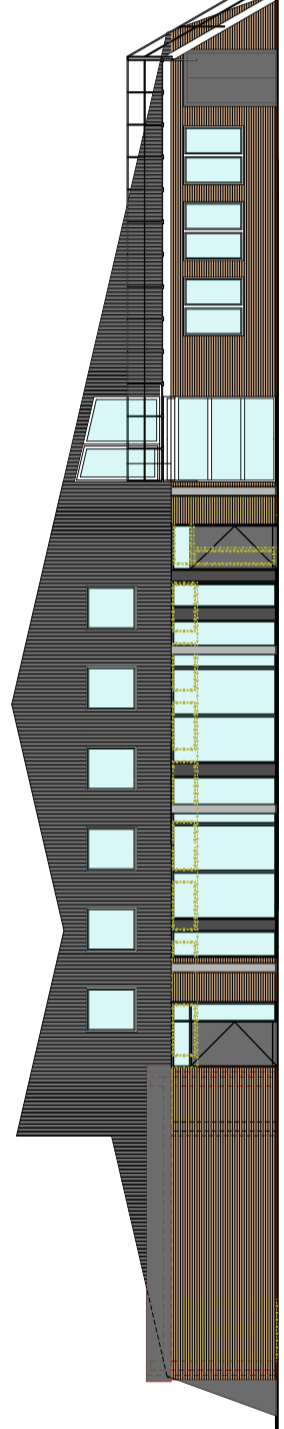
Ansicht Nord
